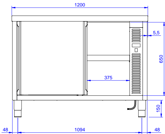
Zepředu
